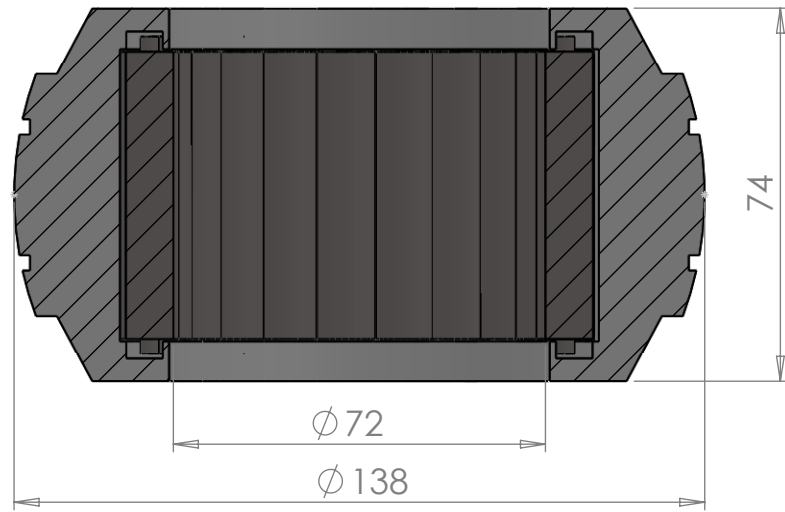
SECTION A-A SCALE 1 : 1.5
