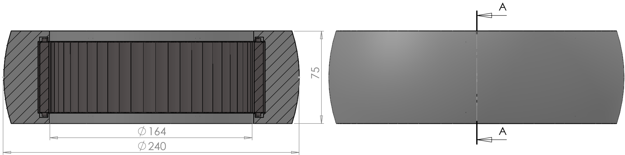
SECTION A-A SCALE 1 : 1.9
