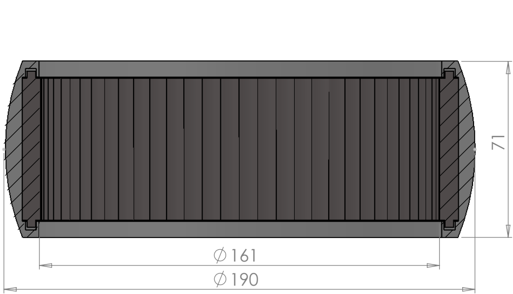
SECTION A-A SCALE 1 : 1.5
