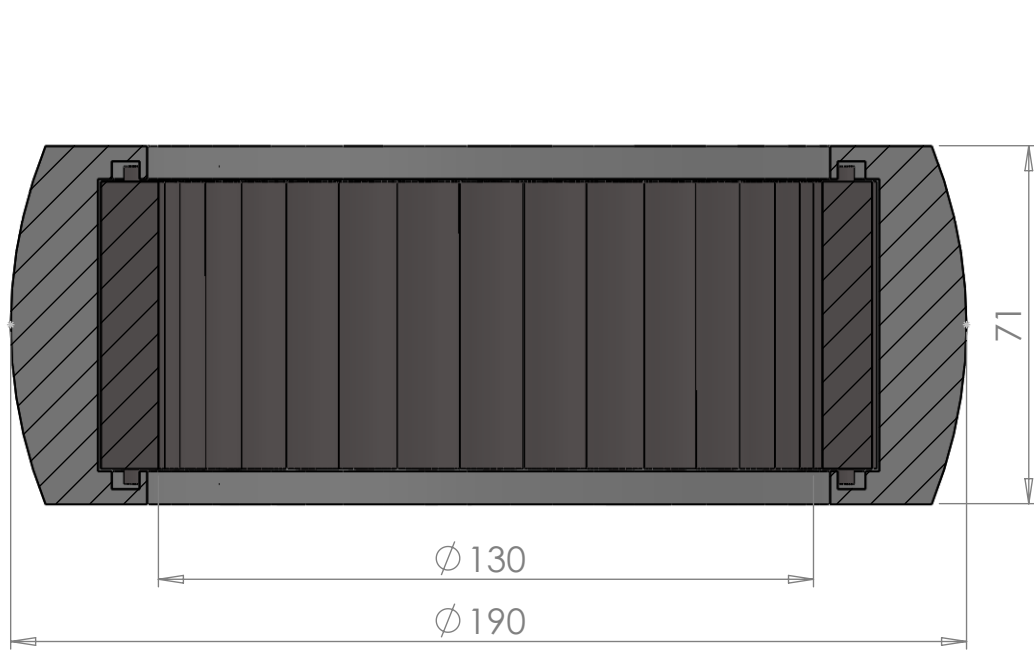
SECTION A-A SCALE 1 : 1.5
