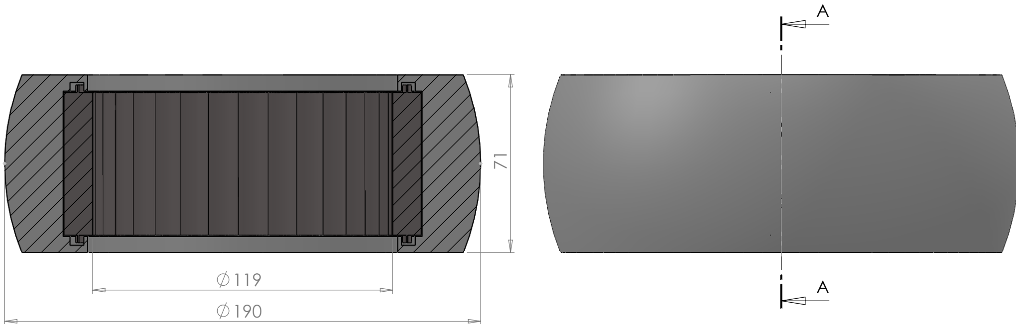
SECTION A-A SCALE 1 : 1.5
