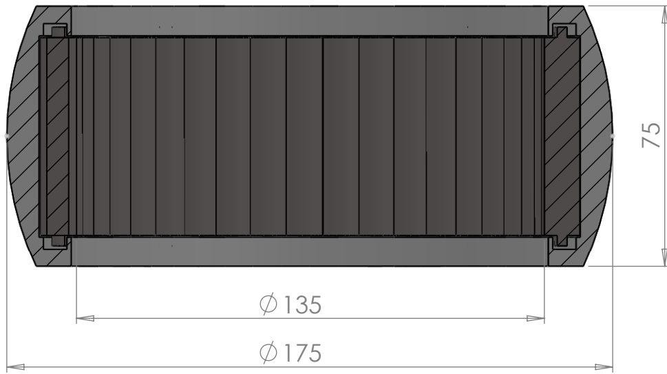
SECTION A-A SCALE 1 : 1.5
