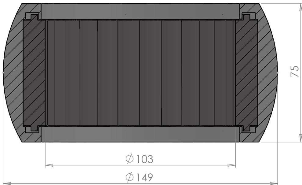
SECTION A-A SCALE 1 : 1.25
