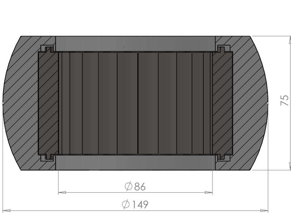
SECTION A-A SCALE 1 : 1.25
