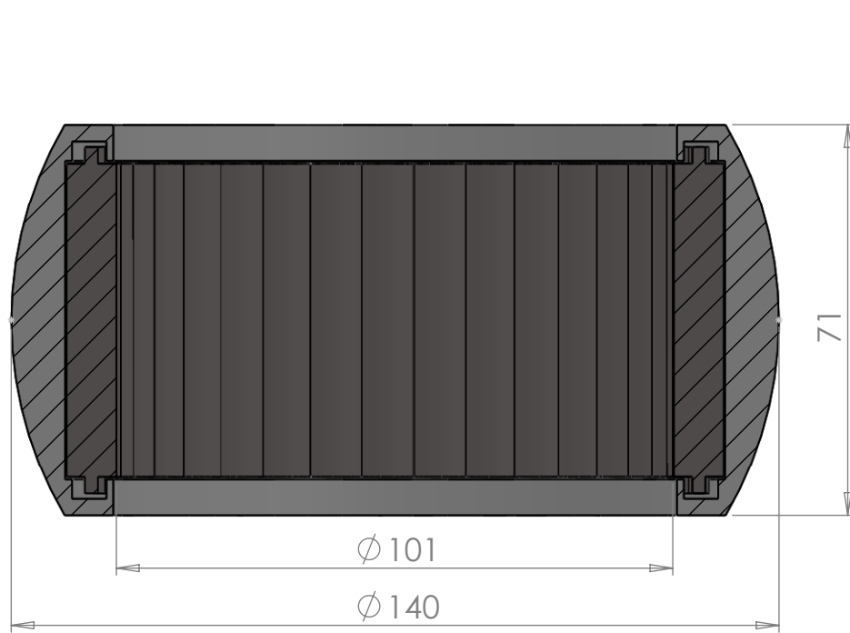
SECTION A-A SCALE 1 : 1.25
