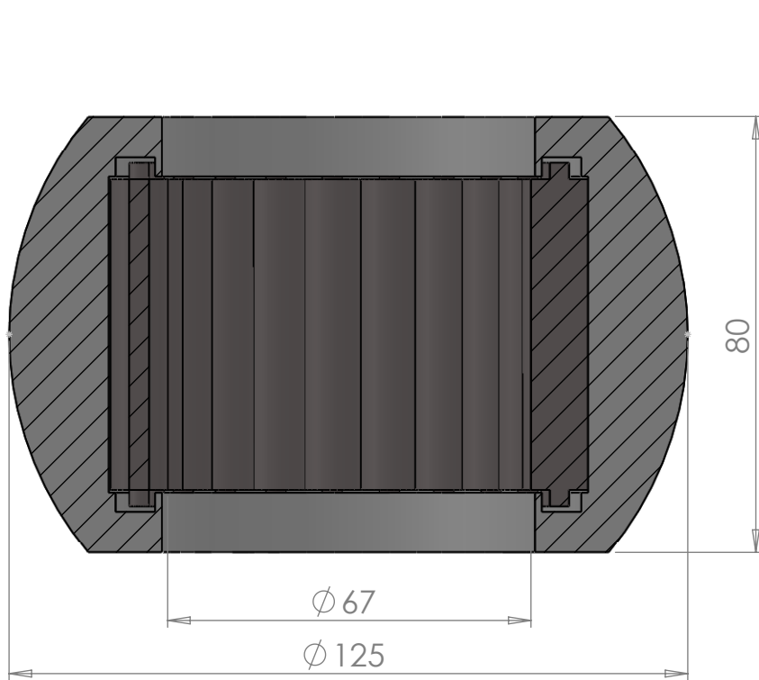
SECTION A-A SCALE 1 : 1.25
