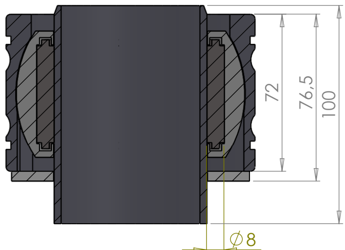
SECTION A-A SCALE 1 : 1.75
