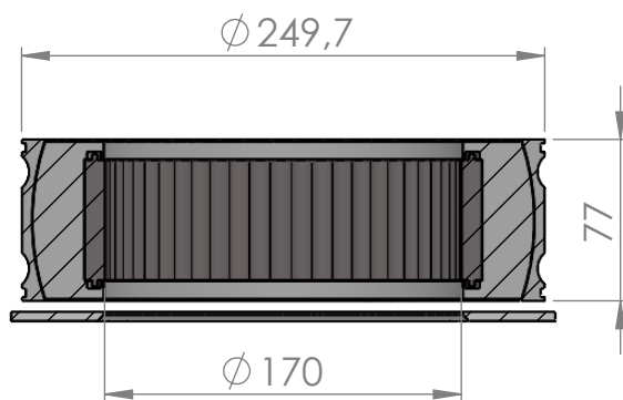
SECTION A-A SCALE 1 : 4
