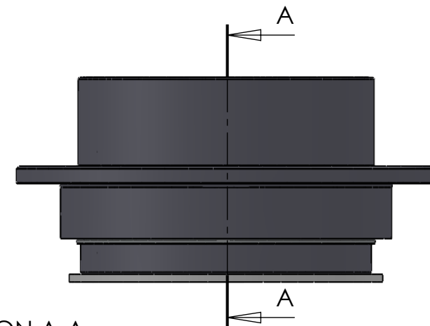
SECTION A-A SCALE 1 : 3
