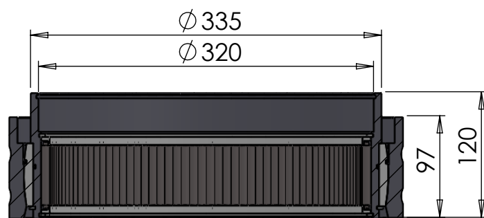
SECTION A-A SCALE 1 : 5
