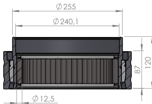
SECTION A-A SCALE 1 : 5
