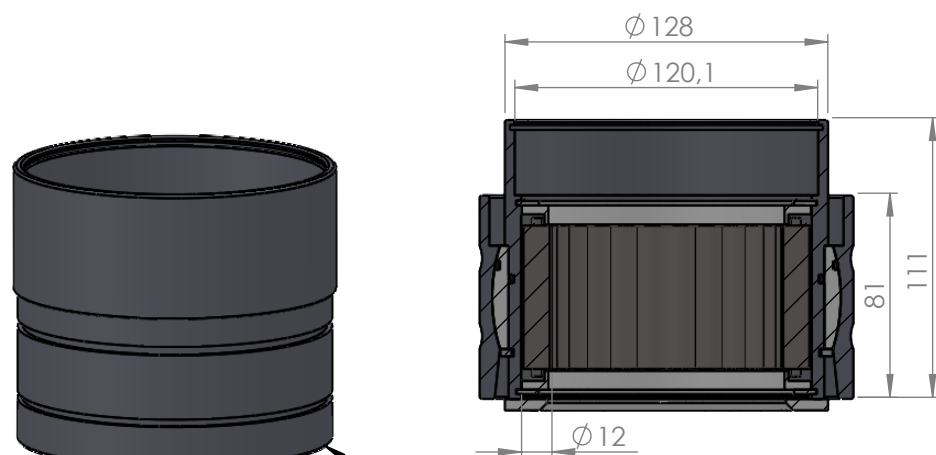
SECTION A-A SCALE 1 : 3
