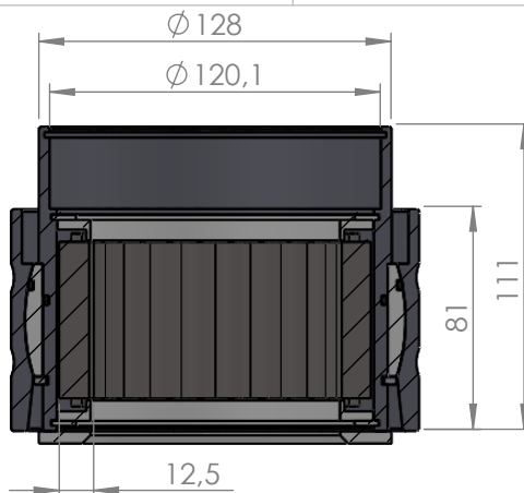
SECTION A-A SCALE 1 : 3
