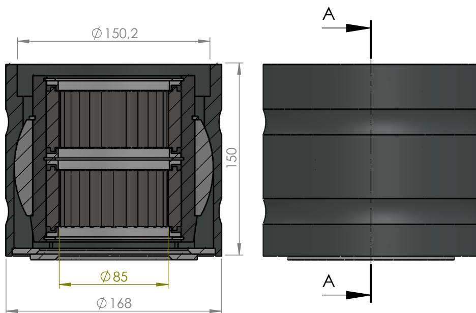
SECTION A-A SCALE 1 : 3
