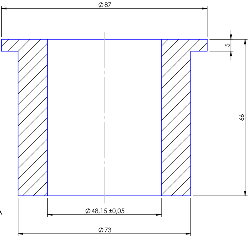
SECTION A-A
